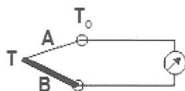
Fig. 2 Simbolizarea termocupurilor
