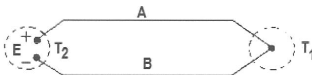
Fig. 1 Structura termocuplului
